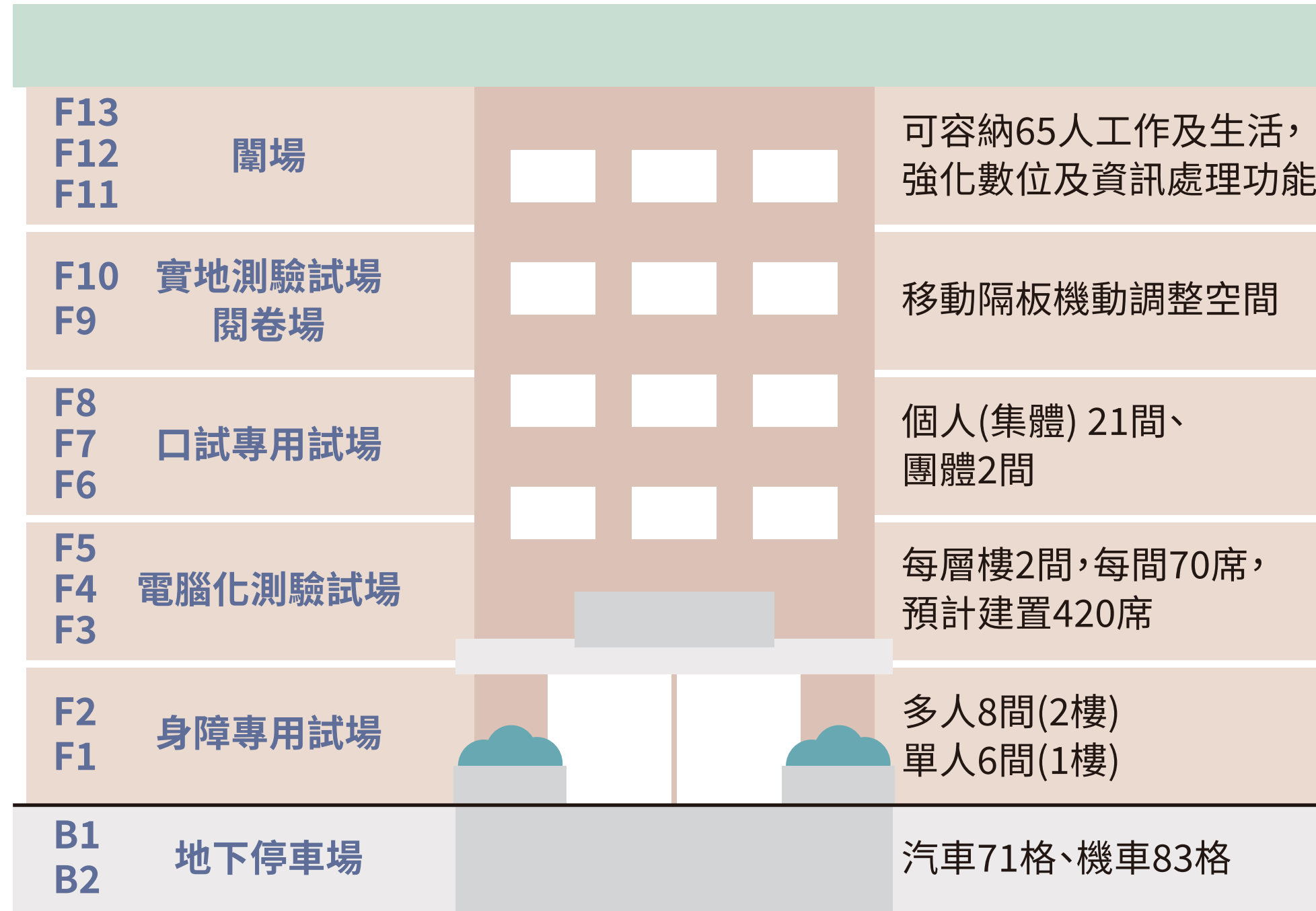
圖3 數位多功能大樓樓層分布
